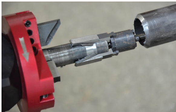
Mandrino piccolo, diametro interno 25 - 32 mm (1" - 1-1/4") Codice prodotto: TRZ-0472-21-00-00-0
